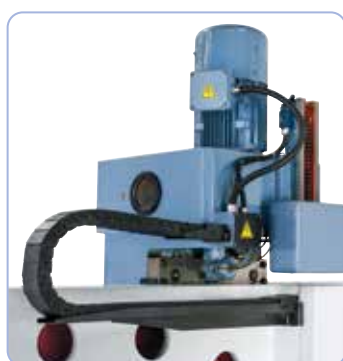
Contrappeso per il mandrino e la catena di conduzione dell'energia nella parte posteriore del portapunta
